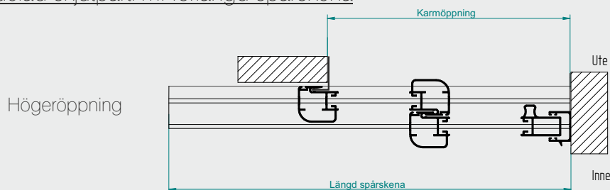
2-delad skjutparti m. förlängd spårskena
